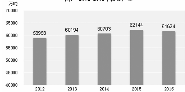
图9 2012-2016年粮食产量
