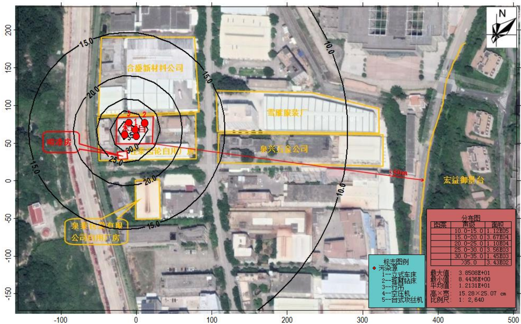
图 4-1 噪声贡献值等值线图
