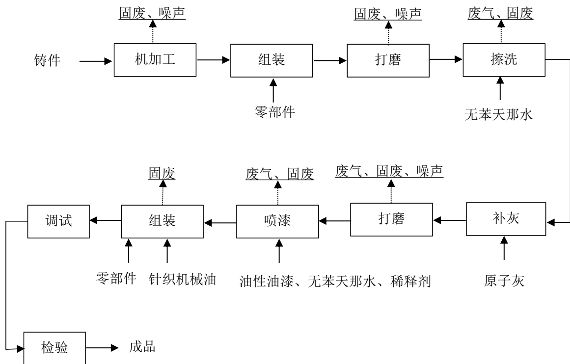
图 3-1 大圆机生产工艺流程图
