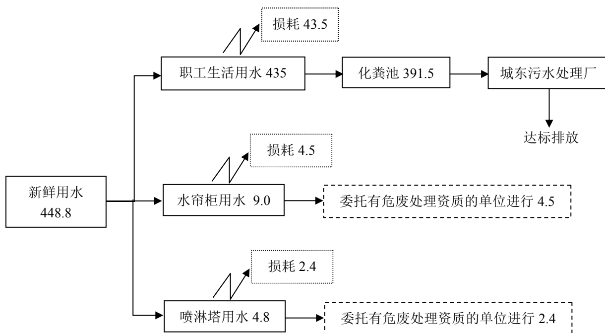
图 3-2 项目水平衡图
