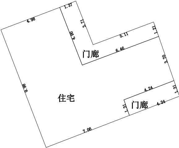
一层平面图
