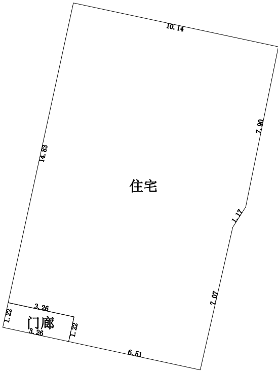
一层平面图
