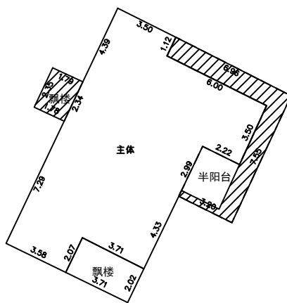
第2层平面图
