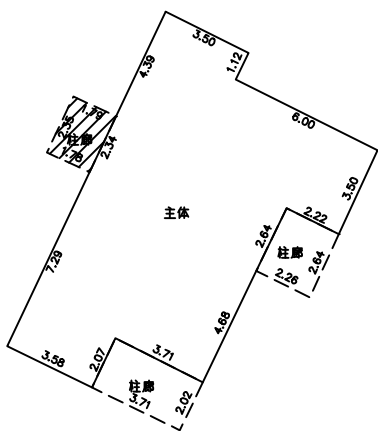
第1层平面图
