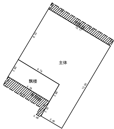
第2层平面图
