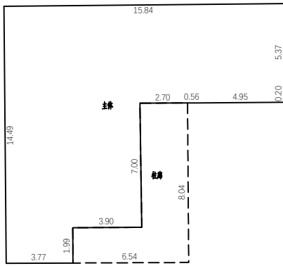
1层平面图
