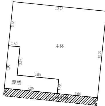
2层平面图
