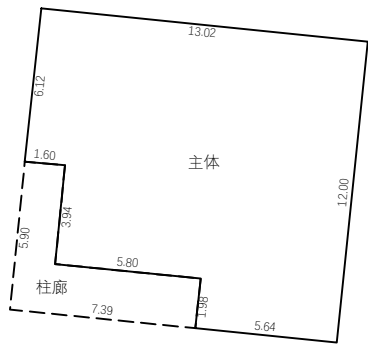
1层平面图
