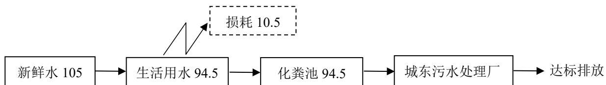
图 3-2 水平衡图
