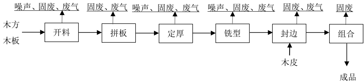
图 3-1 木制家具加工工艺流程图
