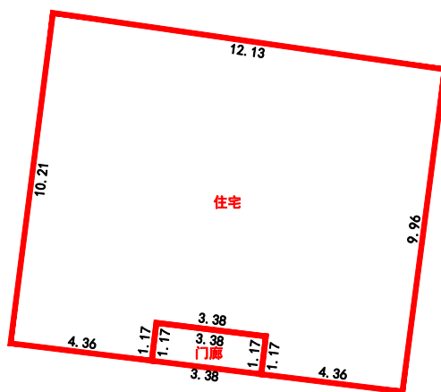
1层平面图
