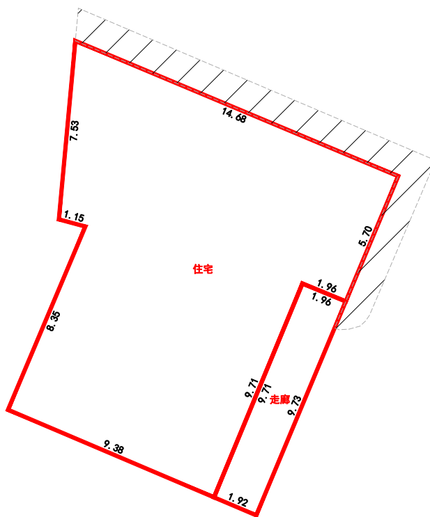
1层平面图
