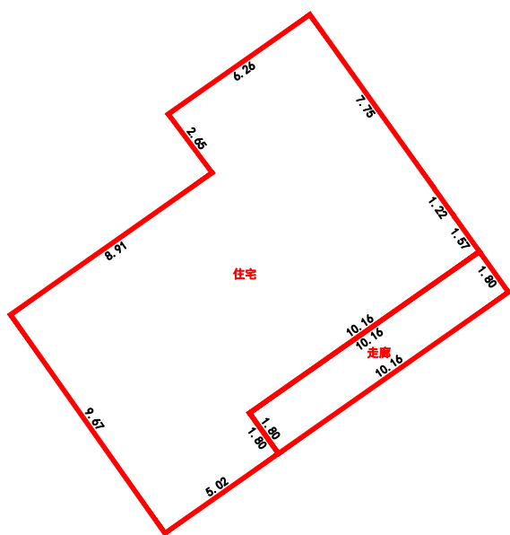
1层平面图
