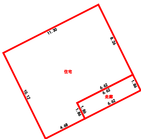
1层平面图
