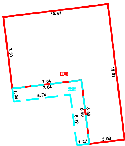
1层平面图
