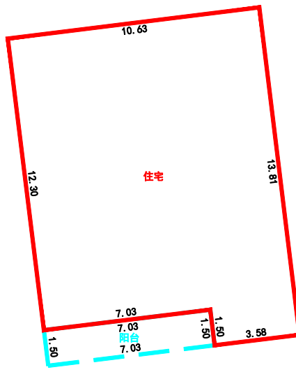
2层平面图
